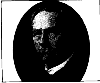
كارل بنتز
