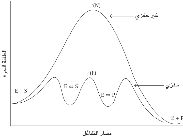
شكل ٦-٣: تمثيل بياني لمسار التفاعل يُبيِّن انخفاض الحاجز بالنسبة إلى خطوة التحوُّل الكيميائي (المحدّدة) للتعامل اللاإنزيمي \ddagger(N) مقابل التفاعل الإنزيمي \ddagger(E) .
