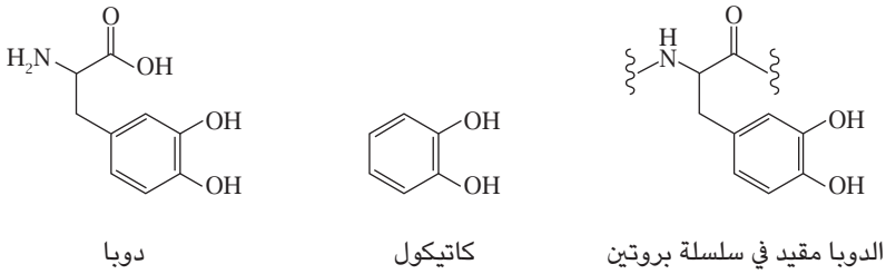
شكل ١٣-٤: جُزء واحد من الدوبا، كاتيكول، والدوبا مُقَيَّد في سلسلة بروتين.
