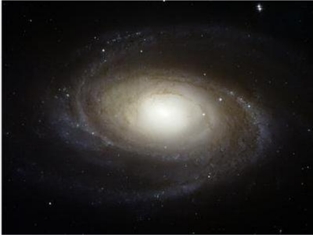
صورة للمجرة البيضاوية
