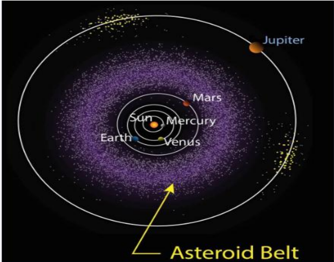
صورة توضح حزام الكويكبات
