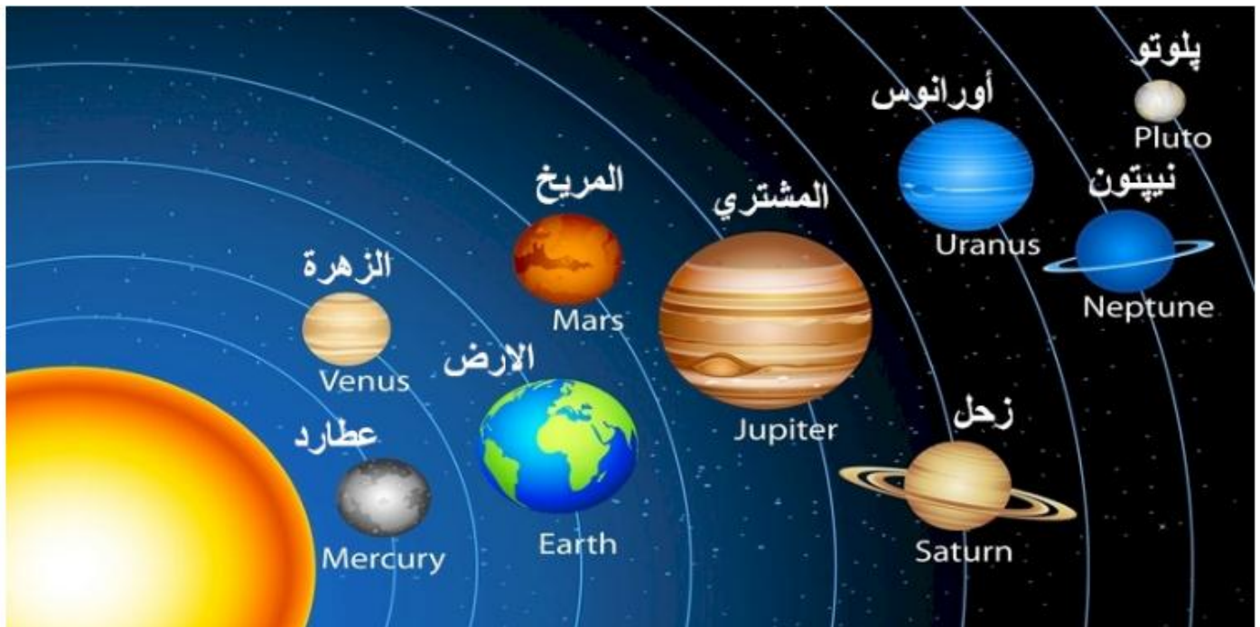
صورة لنظام مجموعتنا الشمسية
