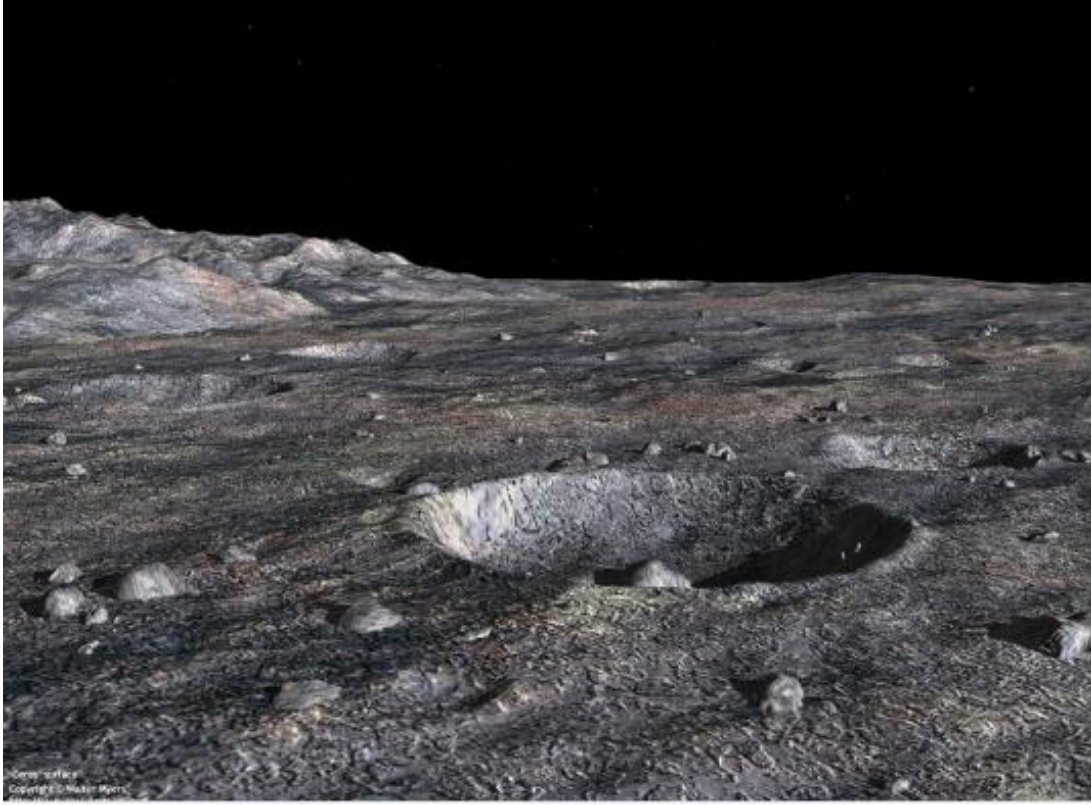
صورة تبين سطح القمر
