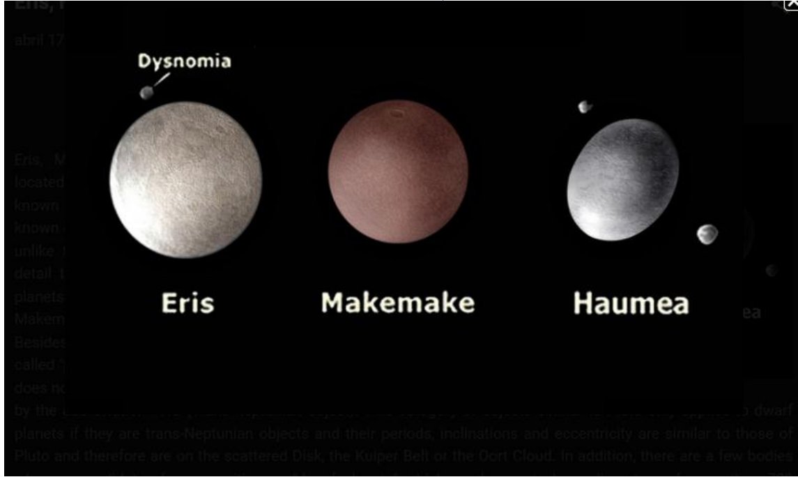
صورة توضح الكواكب القزمة المكتشفة
