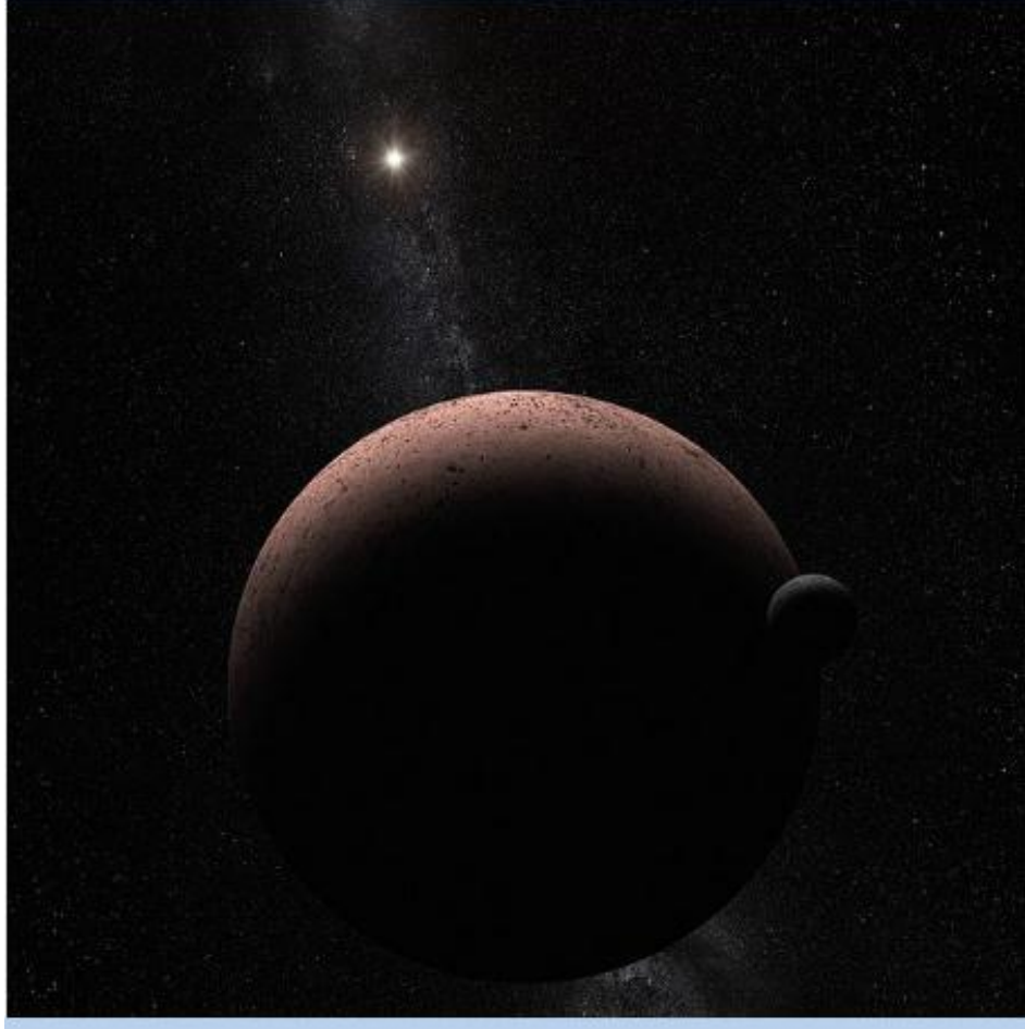
صورة توضح قمر الكوكب القزم ماكيمائي
