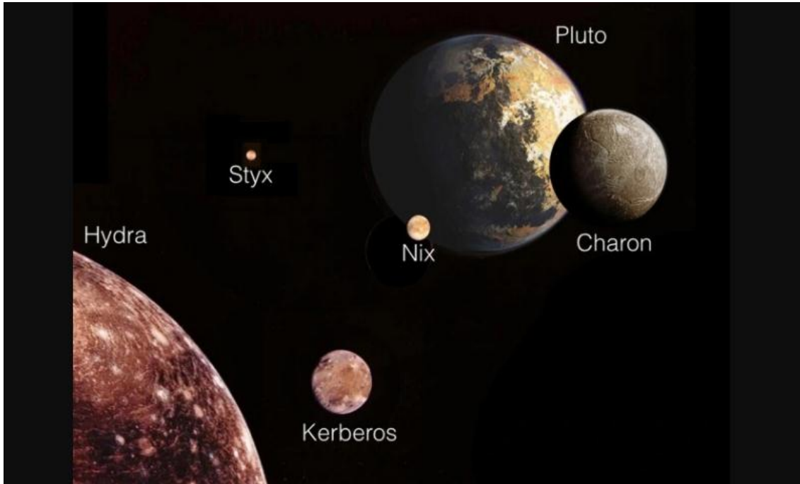
صورة توضح أقمار كوكب بلوتو
