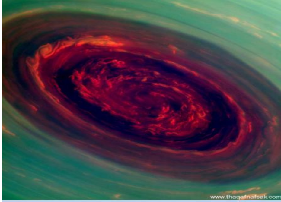
صورة لإعصار ضخم على كوكب زحل
