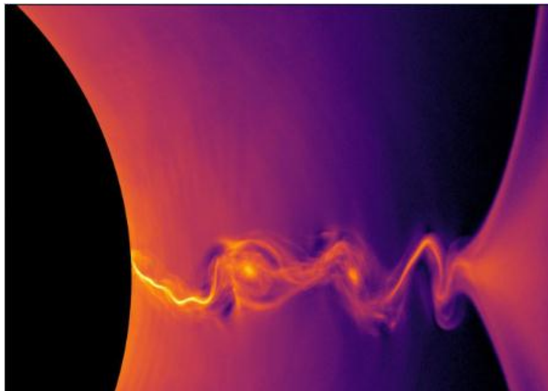
صورة تقريبية لأفق الحدث
